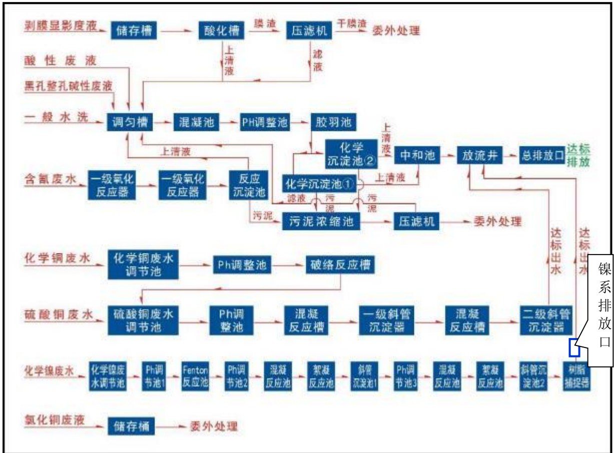
图 2.8.1 废水分质分流处理工艺流程
